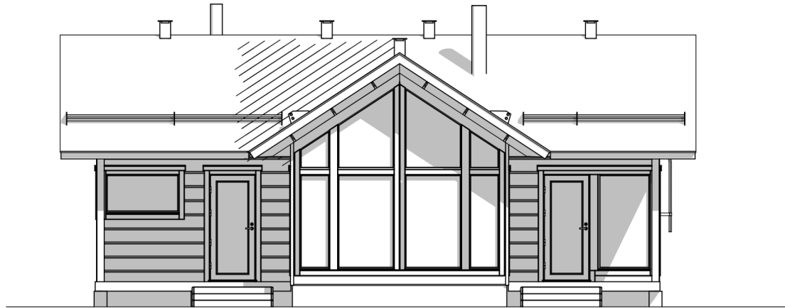
Julkisivu 1 1:100
