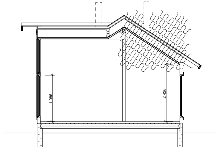
Leikkaus B-B 1:100
