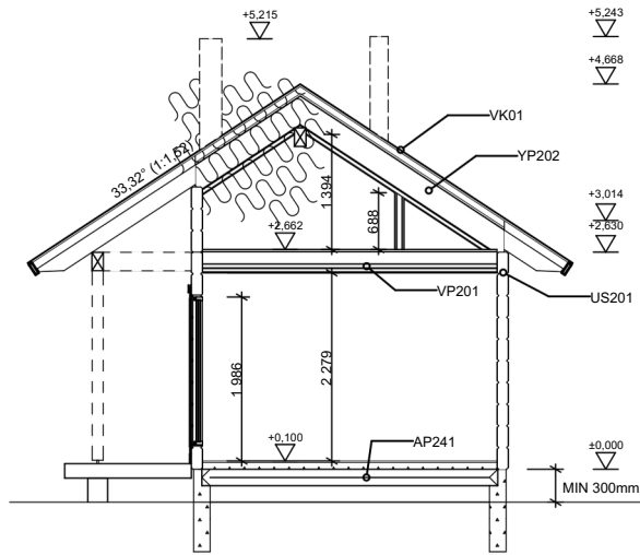
Leikkaus A-A 1:100
