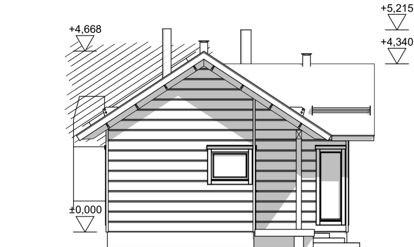
Julkisivu 3 1:100
