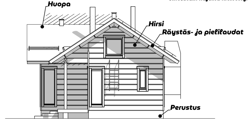
Julkisivu 2 1:100
