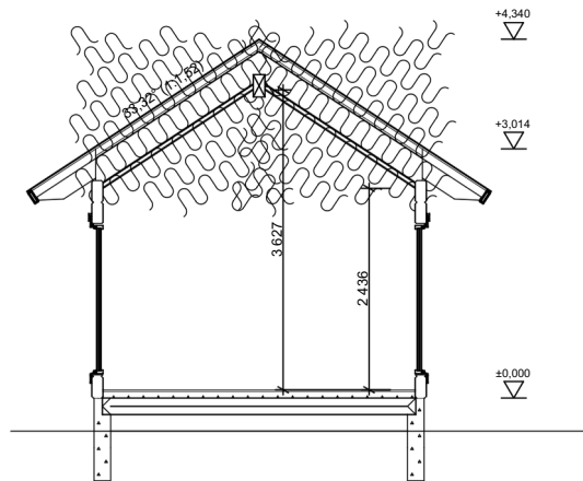
Leikkaus C-C 1:100
