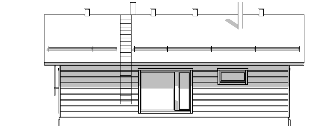
Julkisivu 4 1:100
